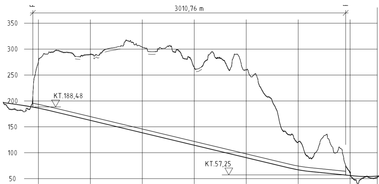
Figur 5. Lengdeprofil Eikeråsheiatunnelen.
