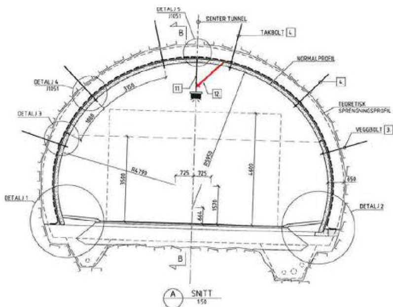
Figur 7.9 Skisse av betongelementhvel, T10,5 [63]
