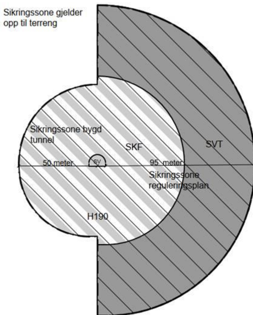
Figur 2. Viser prinsippkisse av tunnel slik den reguleres (høyre halvdel) og slik den tilpasses ferdigstilt samferdselsanlegg (venstre halvdel). (Kilde: Sweco Norge). H190=hensynssone 190. SKF= SVT=
