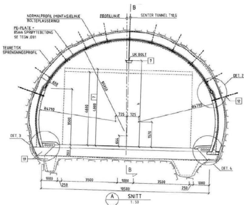
Figur 7.8 Skisse av PE-hvel i heng og med betongelementer i vegg, T10,5 [63]
